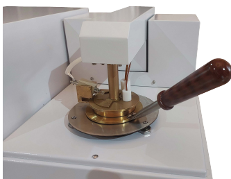
Detalhe - vaso fechado
